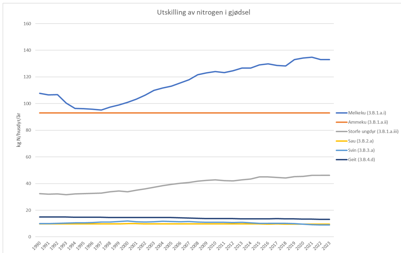
Figur 14 Utskilling av nitrogen i gjødsel per dyr og år i perioden 1990-2023 for melkeku, ammeku, storfe ungdyr, sau, svin og geit. Kg N/husdyr/år. For ammeku bruker vi en konstant nasjonal verdi basert på norske fôrdata tilgjengelig bare for et enkelt år. Kode for utslippskilde er kode i rapporteringen til FN.
