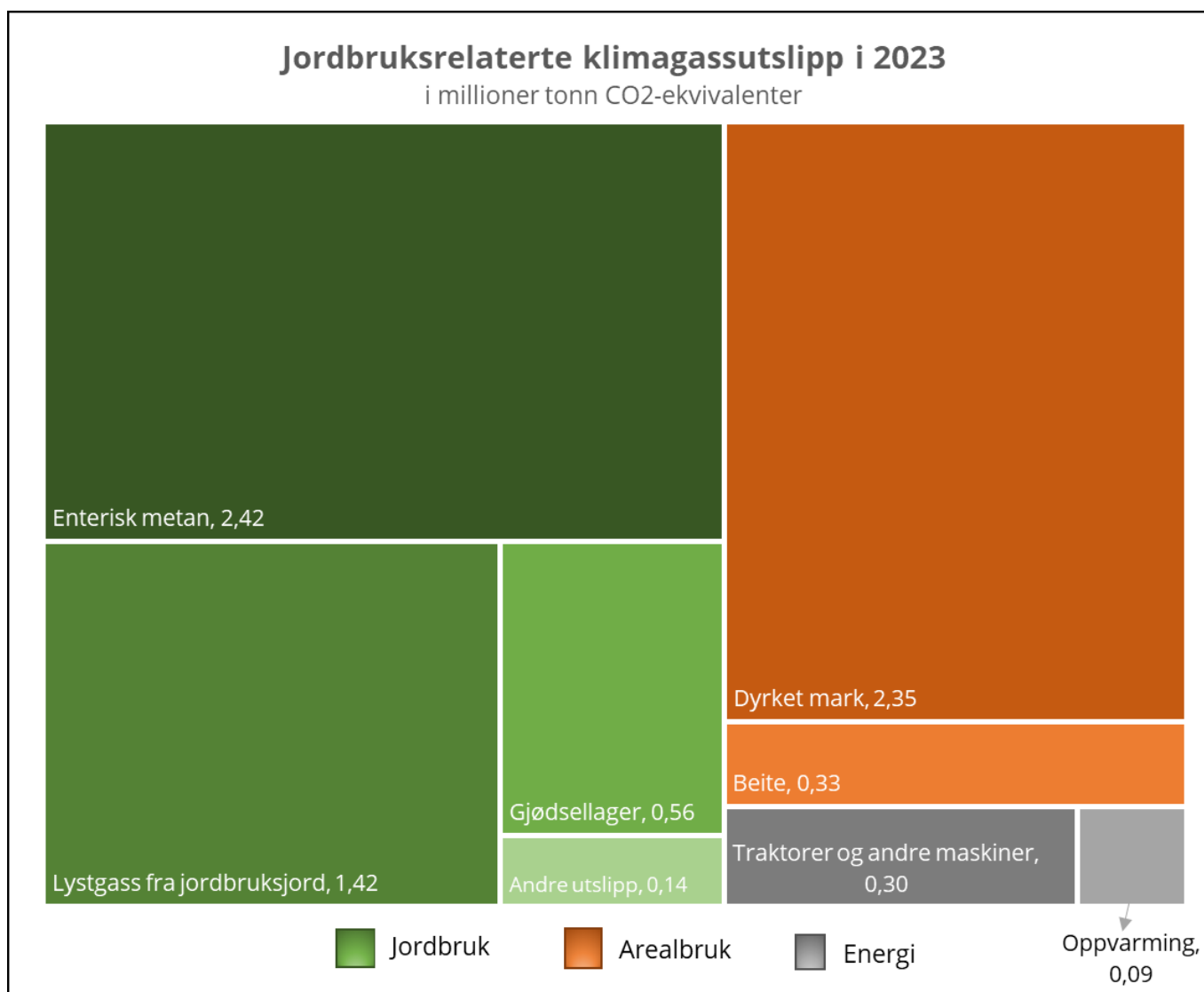
Figur 3 Klimagassutslipp relatert til jordbruket i 2023 fra jordbrukssektoren, energisektoren og arealbrukssektoren. Millioner tonn CO 2 -ekvivalenter.
