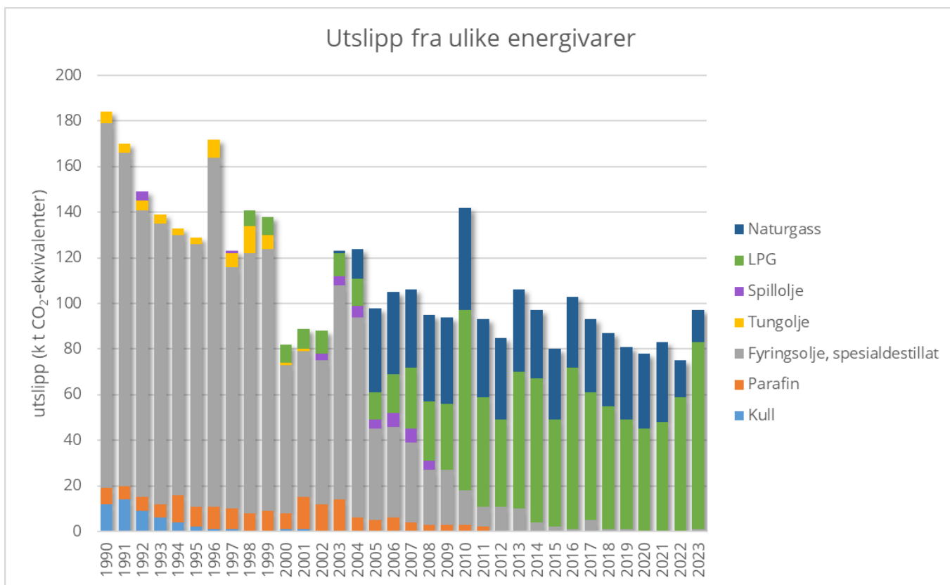
Figur 21 Utslipp i perioden 1990-2023 fra oppvarming med ulike energivarer i primærnæringene. 1000 tonn CO 2 -ekvivalenter. (Kilde: SSB 7 )
