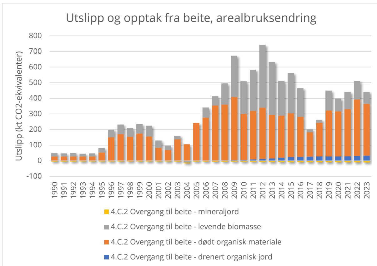
Figur 27 Utslipp og opptak i perioden 1990-2023 fra arealbruksendringer til beite. I 1000 tonn CO 2 -ekvivalenter. Merk at kilde 4.C.2 Overgang til beite – drenert organisk jord er den samme kilden som i Figur 28. Utslippene fra dødt organisk materiale og levende biomasse rapporteres det året en arealbruksendring skjer, og disse vil dermed variere en del fra år til år. Utslipp fra drenert organisk jord fordeler seg over mange år, og variasjonen er dermed mindre. Utslipp fra drenert organisk jord for arealer i overgang til beite er en relativt ny kilde. Det er et lite opptak i mineraljord for arealer i overgang til beite. Kode for utslippkilde er kode i rapporteringen til FN.
