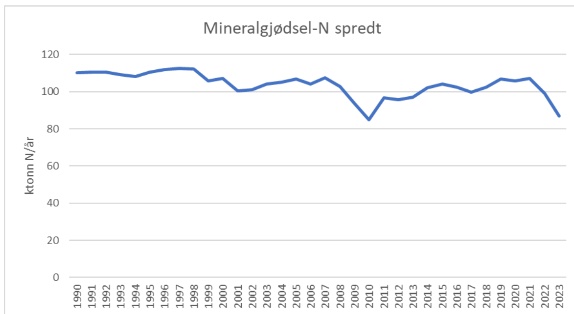
Figur 17 Mineralgjødningnitrogen spredt på jordbruksjord (dyrket mark og beite) i perioden 1990-2023. Kt/yr nitrogen/år.
