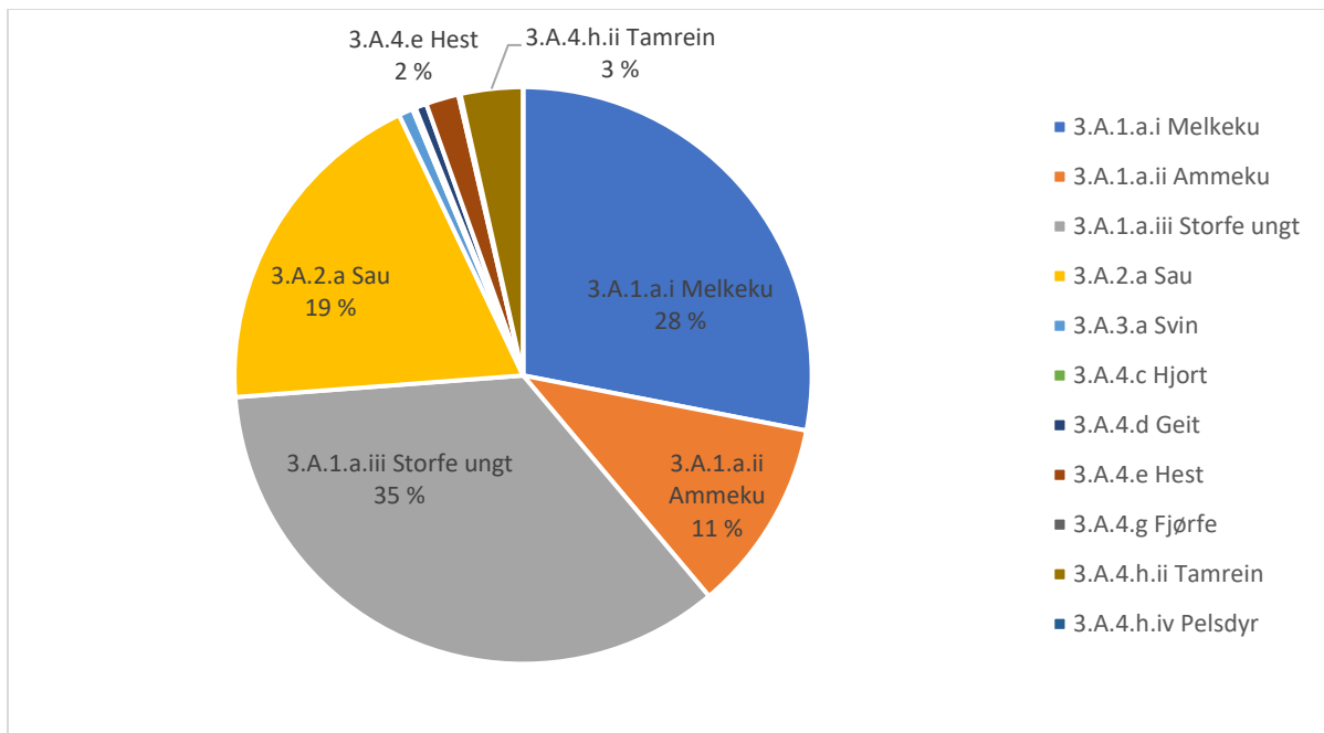
Figur 8 Utslipp av enterisk metan i 2023 fordelt på dyr. Ulike grupper storfe står for rundt 74 prosent av utslippene. Kode for utslippskilde er kode i rapporteringen til FN.
