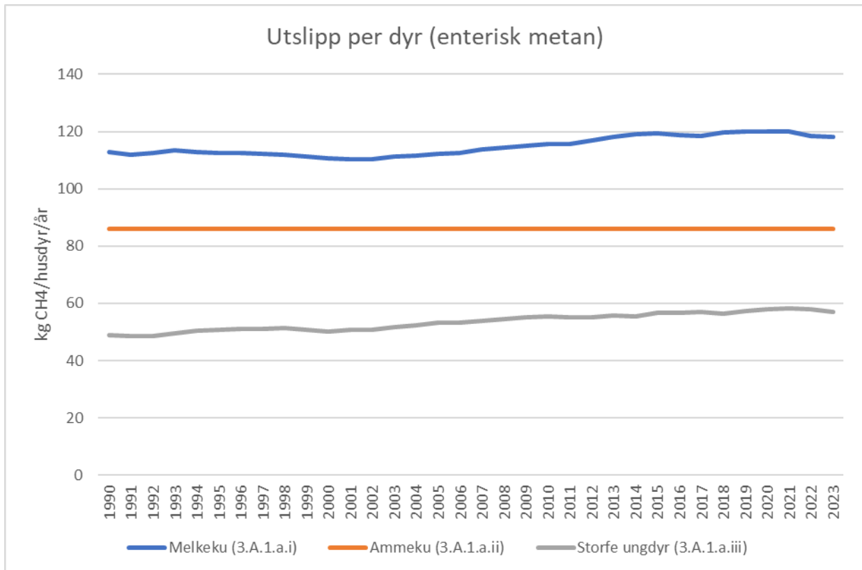
Figur 10 Utslipp per dyr for melkeku, ammeku og storfe ungdyr i perioden 1990-2023. Kg CH 4 /husdyr/år. Kode for utslippsskilde er kode i rapporteringen til FN.
