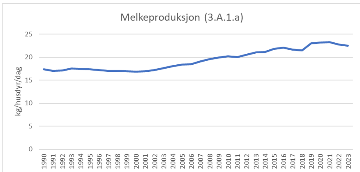
Figur 9 Melkeproduksjon melkeku i perioden 1990-2023. Kg/dag. Kode for utslippskilde er kode i rapporteringen til FN.
