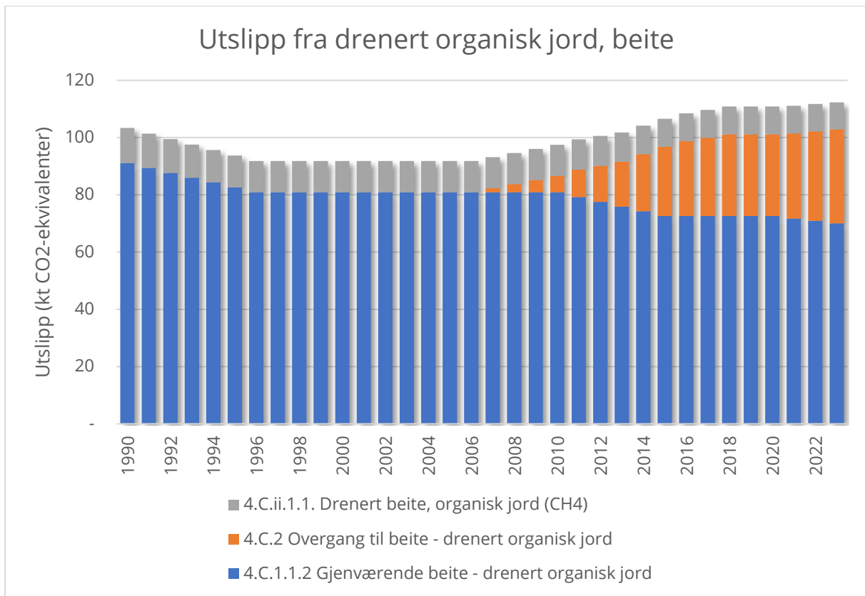
Figur 26 Utslipp i perioden 1990-2023 fra beite på drenert organisk jord. I 1000 tonn CO 2 -ekvivalenter. Kilde 4.C.ii.1.1. omfatter metanutslipp fra drenerte arealer, mens kilde 4.C.2 og 4.C.1.1.2. omfatter CO 2 -utslipp fra nedbrytning av organisk materiale. Kode for utslippskilde er kode i rapporteringen til FN.
