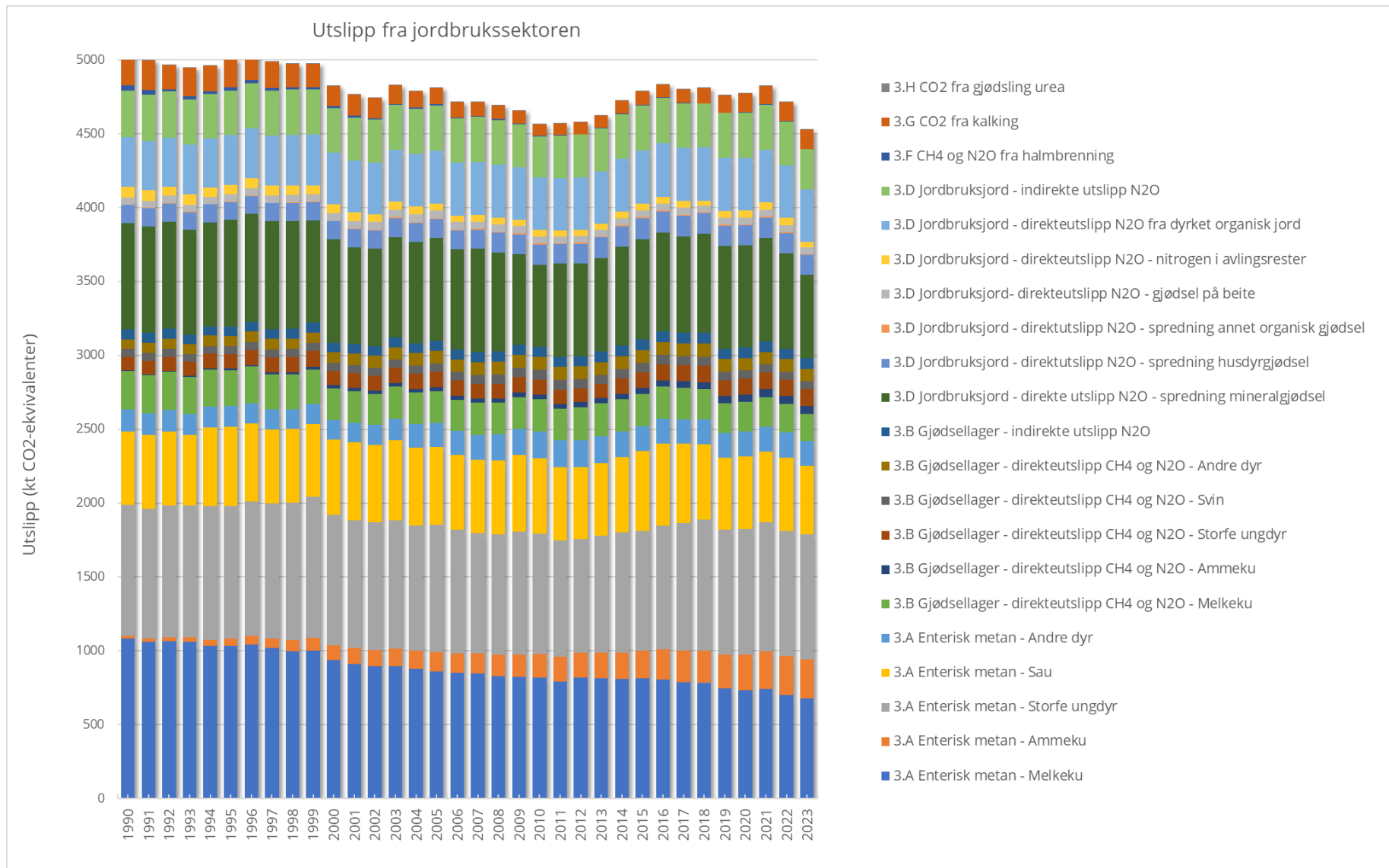
Figur 4 Utslipp 1990-2023 for alle utslippsskilder i jordbrukssektoren (3A-3H), 1000 tonn CO 2 -ekvivalenter. Kode for utslippsskilde er kode i rapporteringen til FN.
