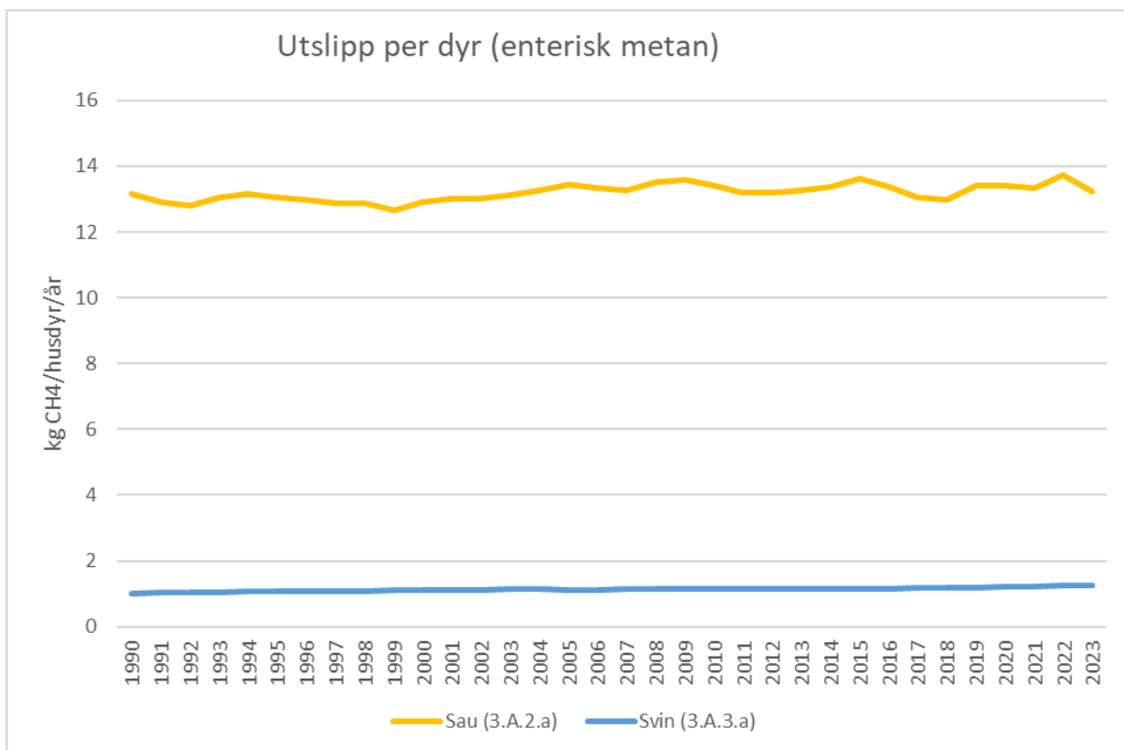
Figur 11 Utslipp per dyr for sau og svin, i perioden 1990-2023. Kg CH 4 /husdyr/år. Kode for utslippsskilde er kode i rapporteringen til FN.
