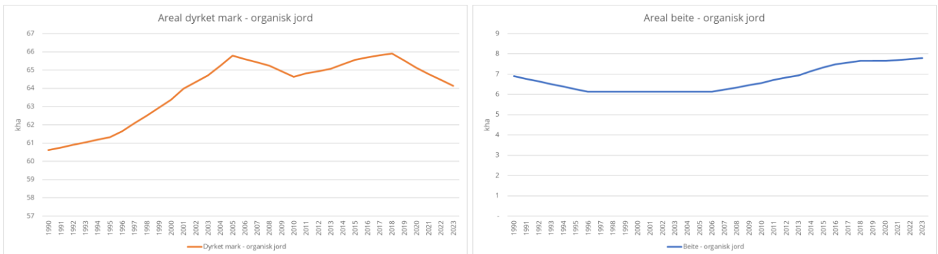
Figur 23 Areal av dyrket mark og beite på organisk jord i perioden 1990-2023, i 1000 hektar. Merk ulike verdier på y-aksen.
