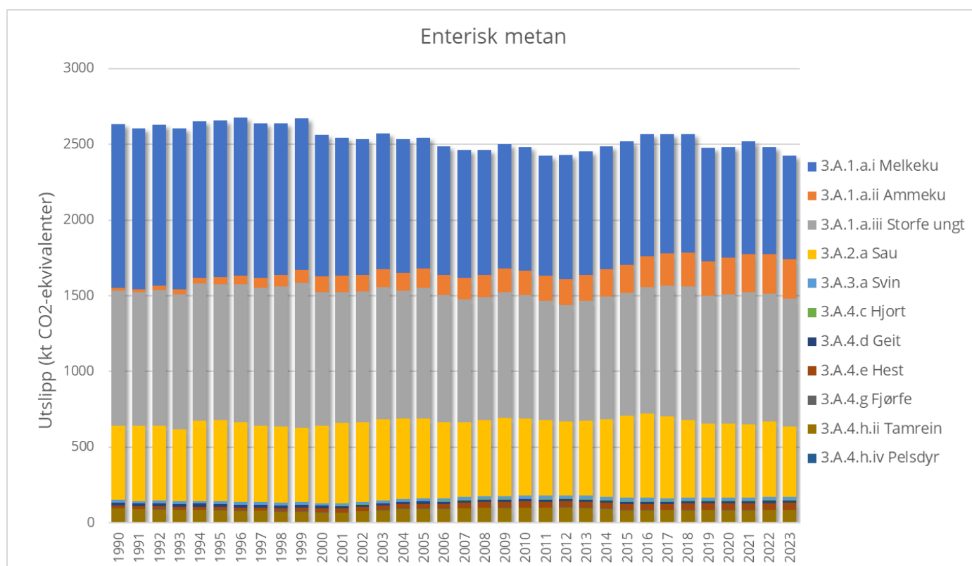
Figur 7 Utslipp av enterisk metan for ulike husdyrgrupper i perioden 1990-2023. I 1000 tonn CO 2 -ekvivalenter. Kode for utslippsskilde er kode i rapporteringen til FN.
