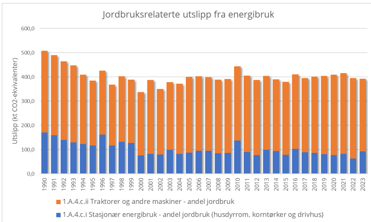
Figur 19 Jordbruksrelaterte utslipp fra energibruk (del av CRT-kilder 1A4ci og -ii) i perioden 1990-2023. I 1000 tonn CO 2 -ekvivalenter. Kode for utslippskilde er kode i rapporteringen til FN.
