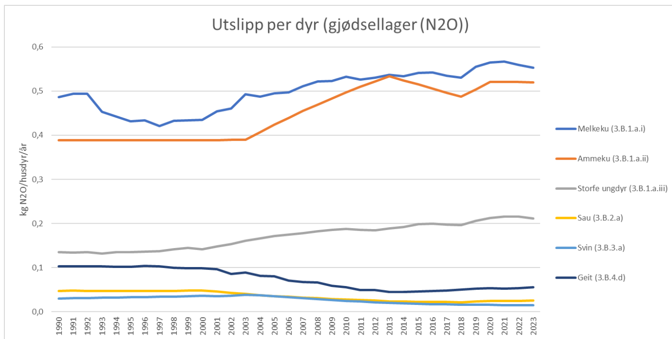
Figur 15 Utslipp per dyr av N 2 O fra gjødsellager i perioden 1990-2023. Melkeku, ammeku, storfe ungdryr, sau, svin og geit. Kg N 2 O/husdyr/år. Kode for utslippkilde er kode i rapporteringen til FN.
