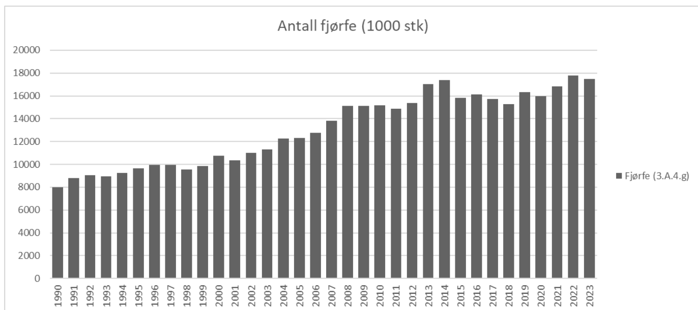
Figur 6 Utviklingstrend for antall fjørfe i perioden 1990-2023. 1000 stk. Kode for utslippskilde er kode i rapporteringen til FN.
