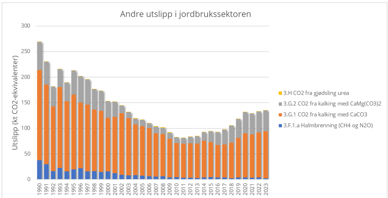
Figur 18 Utslipp fra kalking, halmbrenning og CO 2 utslipp fra gjødsling med urea i perioden 1990-2023. Tonn CO 2 -ekvivalenter. Kode for utslippkilde er kode i rapporteringen til FN.
