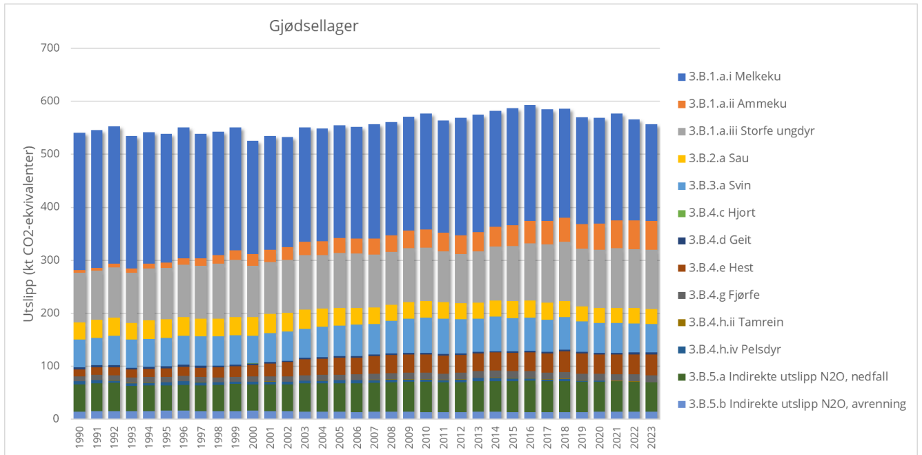
Figur 12 Utslipp av metan og lystgass fra gjødsellager i perioden 1990-2023. Tonn CO 2 -ekvivalenter. Kode for utslippkilde er kode i rapporteringen til FN.
