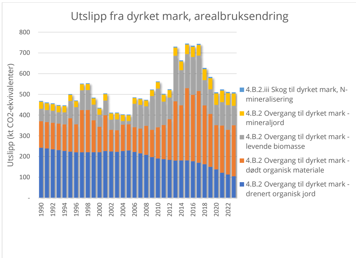
Figur 25 Utslipp i perioden 1990-2023 fra arealbruksendringer til dyrket mark. I 1000 tonn CO 2 -ekvivalenter. Merk at kilde 4.B.2 Overgang til dyrket mark – drenert organisk jord er den samme kilden som i Figur 26. Utslippene fra dødt organisk materiale og levende biomasse rapporteres det året en arealbruksendring skjer, og disse vil dermed variere en del fra år til år. Utslipp fra drenert organisk jord og mineraljord fordeler seg over mange år, og variasjonen er dermed mindre. Utslippene fra drenert organisk jord er nedadgående. Kode for utslippsskilde er kode i rapporteringen til FN.
