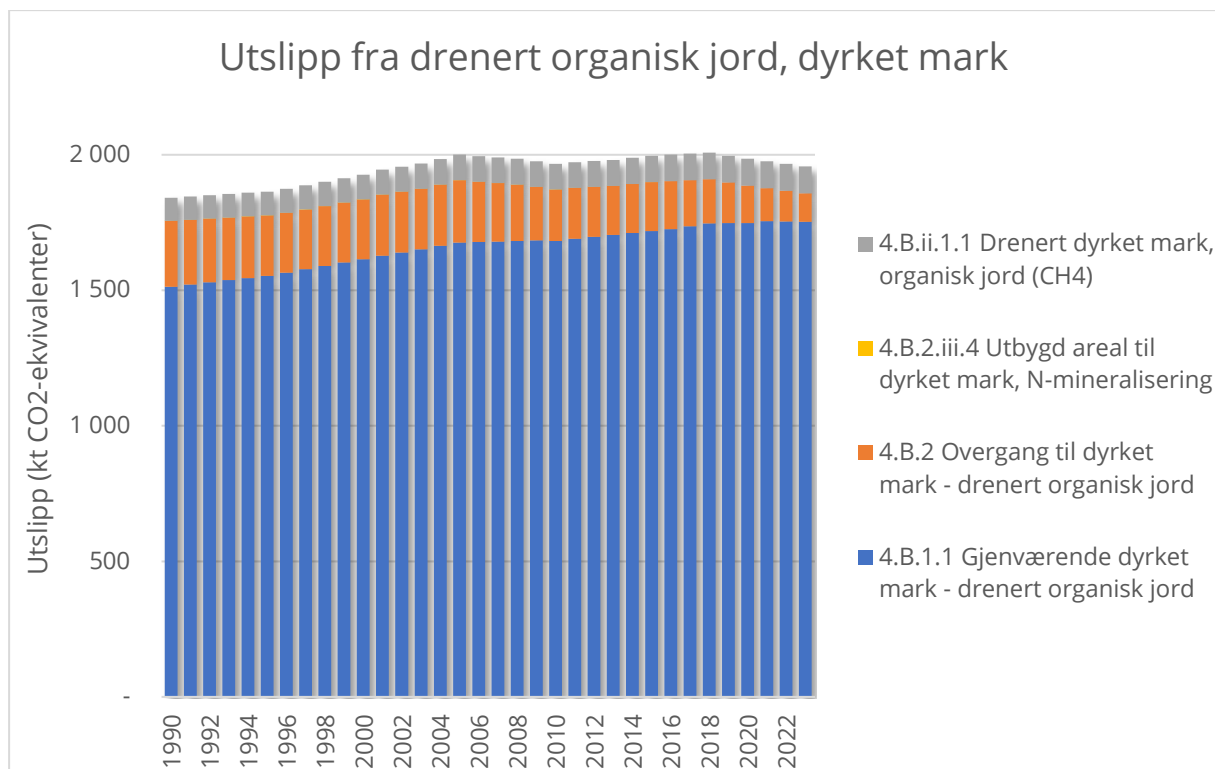
Figur 24 Utslipp fra dyrket mark på drenert organisk jord i perioden 1990-2023. I 1000 tonn CO 2 -ekvivalenter. Kilde 4.B.ii.1.1 omfatter metanutslipp fra drenerte arealer, mens 4.B.iii.4 omfatter lystgassutslipp fra nitrogenmineralisering. Kilde 4.B.2 og 4.B.1.1 omfatter CO 2 -utslipp fra nedbrytning av organisk materiale. Kode for utslippskilde er kode i rapporteringen til FN.
