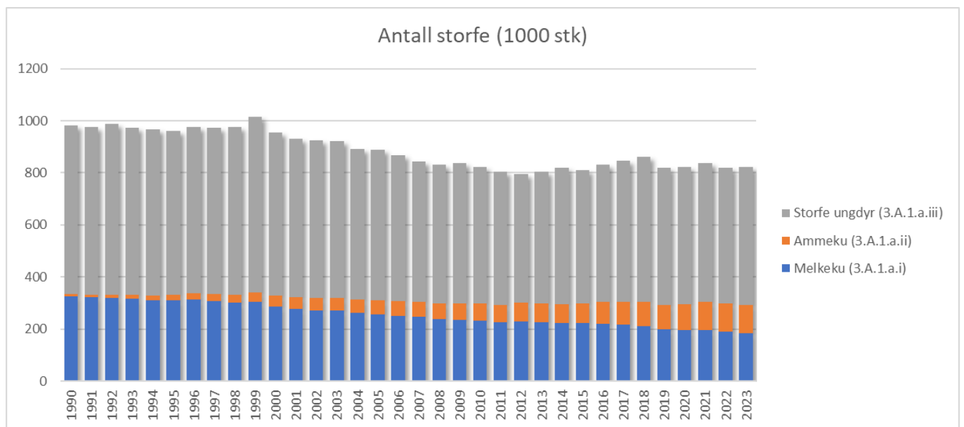
Figur 5 Utviklingstrend for antall storfe 1990-2023 (Melkeku, ammeku, storfe ungdyr). 1000 stk. Kode for utslippskilde er kode i rapporteringen til FN.
