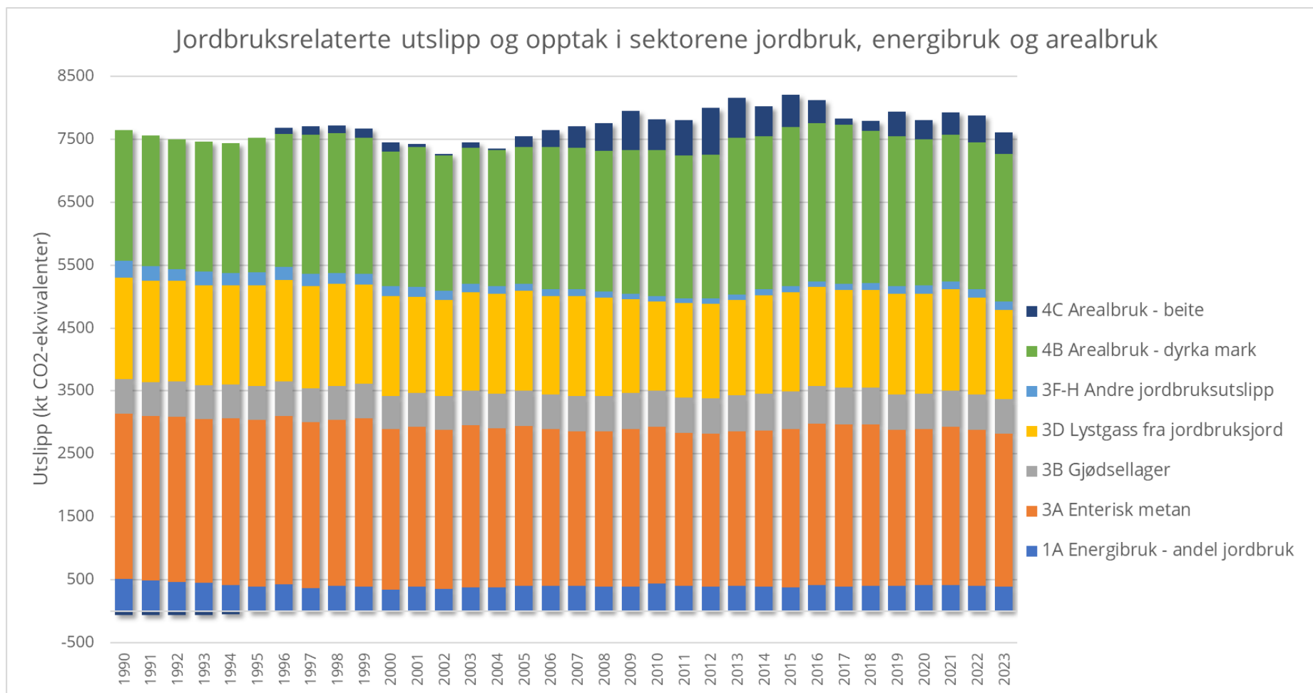
Figur 2 Jordbruksrelaterte utslipp og opptak i sektorene jordbruk, energibruk og arealbruk i perioden 1990-2023 i 1000 tonn CO 2 -ekvivalenter (AR5 3 ). Kode for utslippskilde er kode i rapporteringen til FN.
