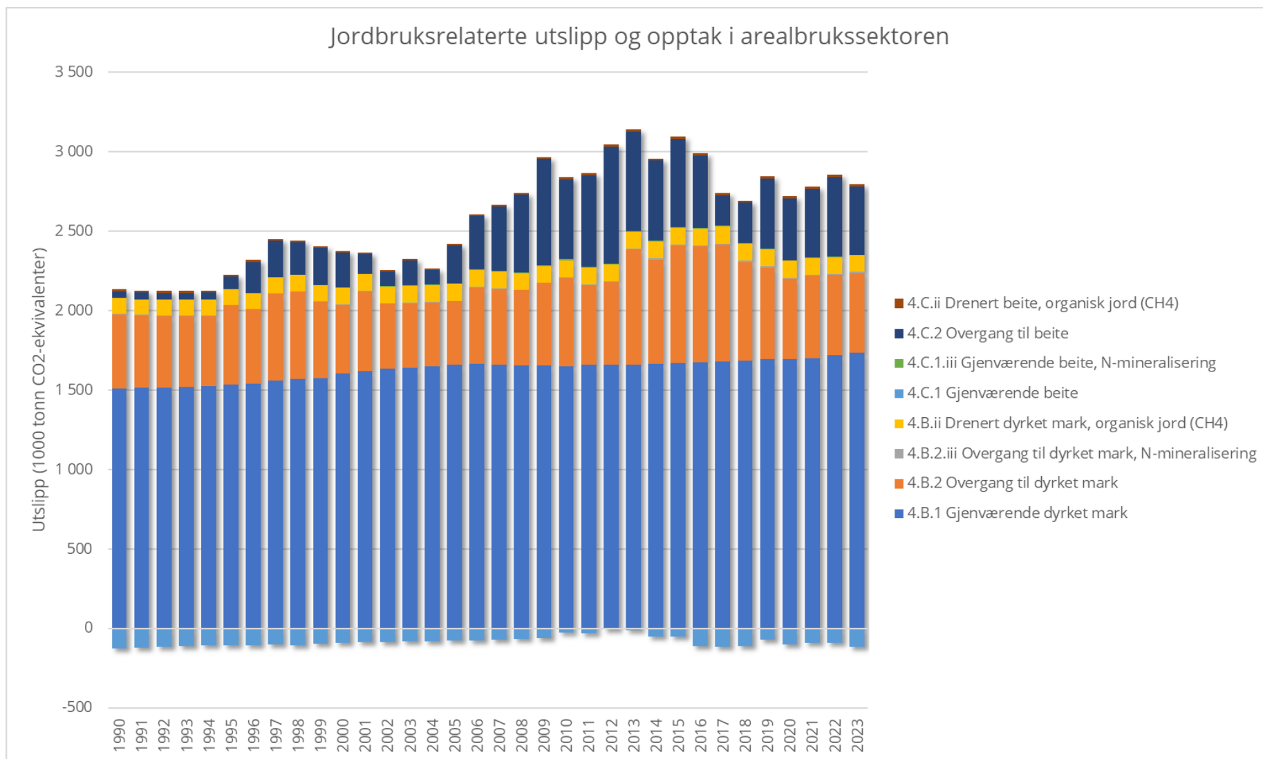
Figur 22 Utslipp i perioden 1990-2023 i 1000 tonn CO 2 -ekvivalenter på detaljert kildenivå for de jordbruksrelaterte arealbrukskildene. Omfatter både CO 2 -utslipp, N 2 O-utslipp fra N-mineralisering, og CH 4 -utslipp fra drenerte arealer. Kode for utslippkilde er kode i rapporteringen til FN.
